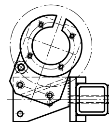
Ansicht D
