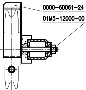
Schnitt A-A
