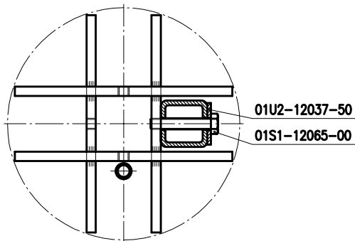
Schnitt B-B
